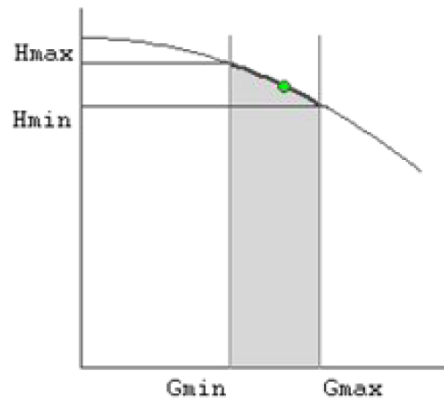
Рисунок 26. Напорно-расходная характеристика насоса
