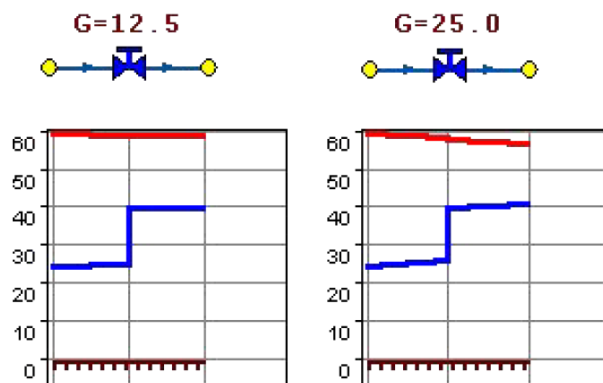
Рисунок 30. Регулятор давления
