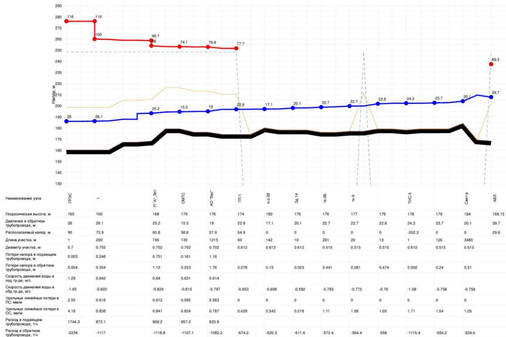
Рисунок 33. Пьезометрический график от Красноярской ГРЭС-2 до АБЗ (1 и 2 очереди).
