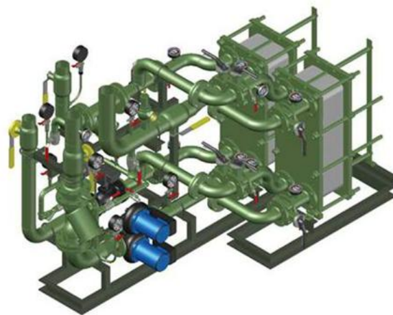
МОДУЛЬ СИСТЕМЫ ОТОПЛЕНИЯ (ВЕНТИЛЯЦИИ) С НЕЗАВИСИМЫМ ПРИСОЕДИНЕНИЕМ, ЧЕРЕЗ ТЕПЛОБМЕННЫЕ АППАРАТЫ (100% РЕЗЕРВИРОВАНИЕ) ПОКАЗАН В СТАНДАРТНОМ ИСПОЛНЕНИИ. БЛОК 100% РЕЗЕРВИРОВАНИЯ ИМЕЕТ ВАРИАНТЫ УСТАНОВКИ, ОТЛИЧНЫЕ ОТ СТАНДАРТНОГО ИСПОЛНЕНИЯ.
