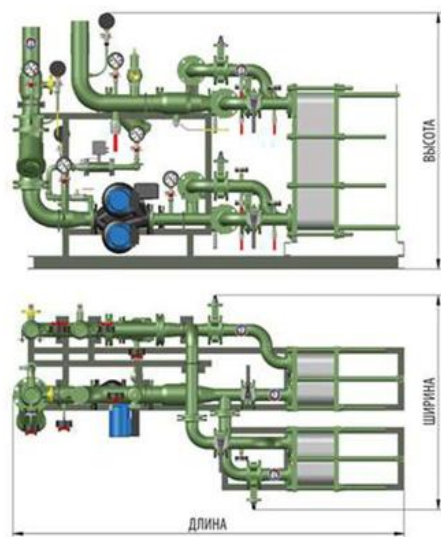
Рисунок 43. Модуль системы отопления с независимым присоединением, через теплообменные
